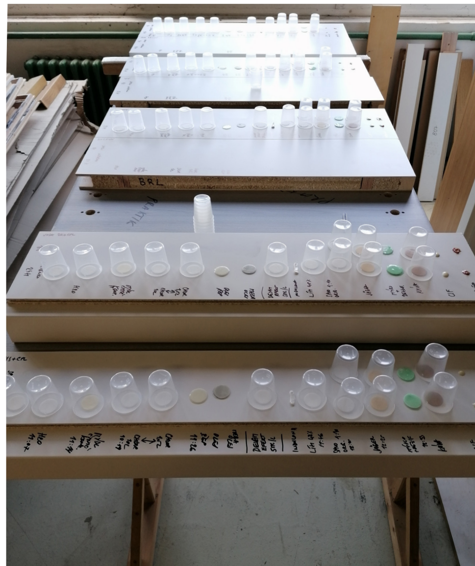
Testování odolnosti povrchu vůči kapalinám a jejich následné čištění.
